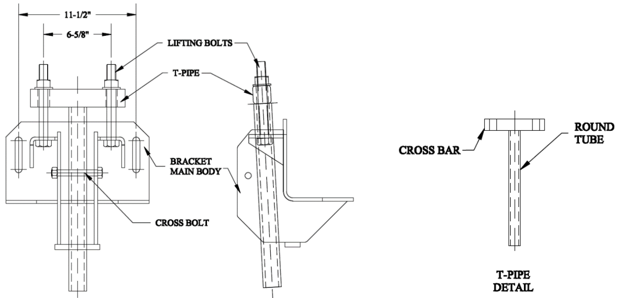
SDB bracket
