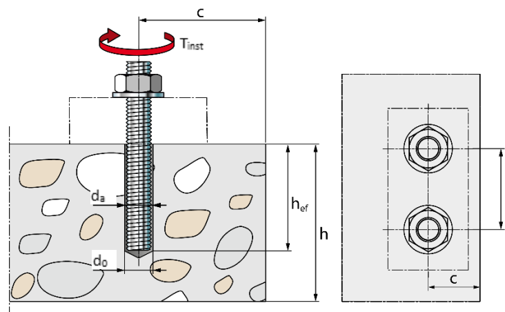
FIGURE 1—INSTALLATION PARAMETERS
