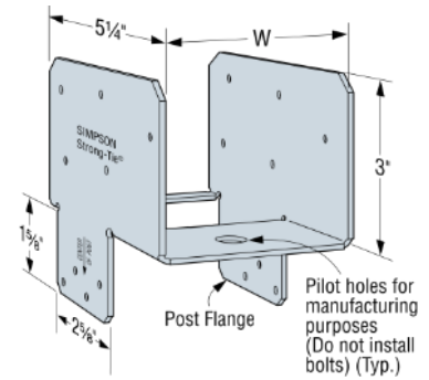
EPCZ End Post Cap
